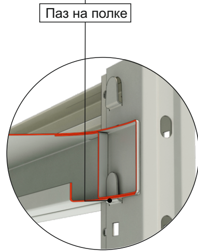
Второй этап- установка и закрепление второй стойки на балках рамных, консольно закрепленных на первой стойке
